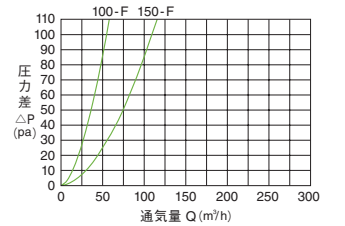
<圧力差-通気量曲線>
